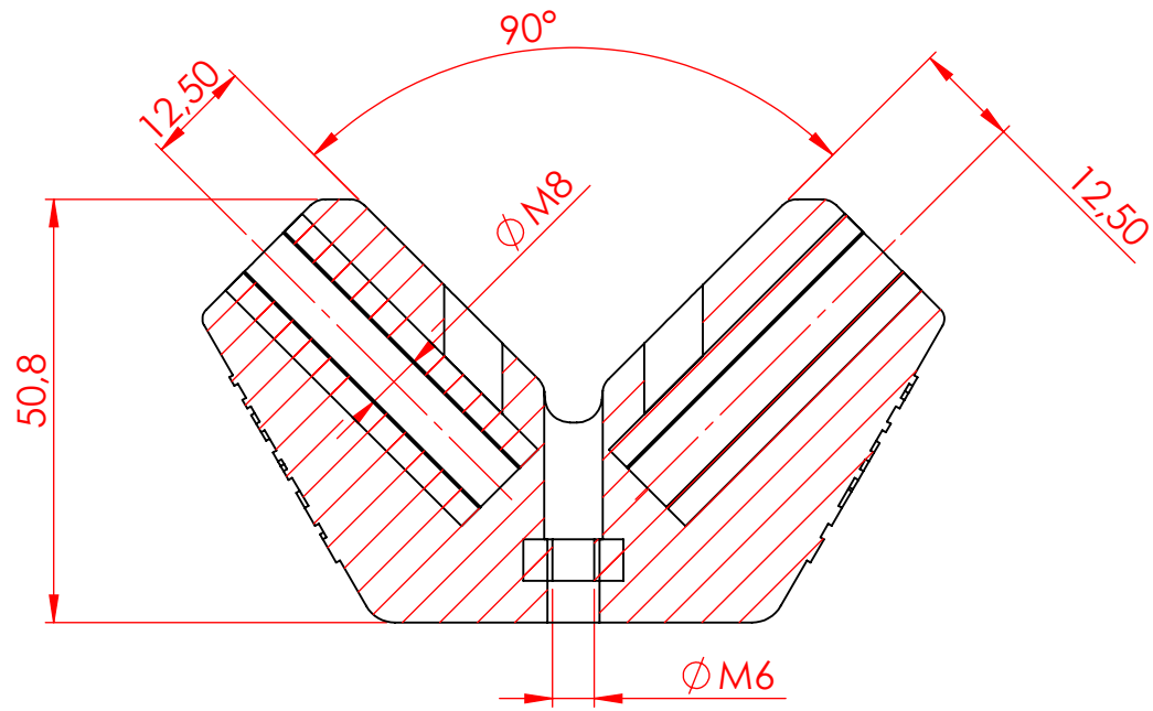
KESIT B-B ÖLÇEK 1 : 1
